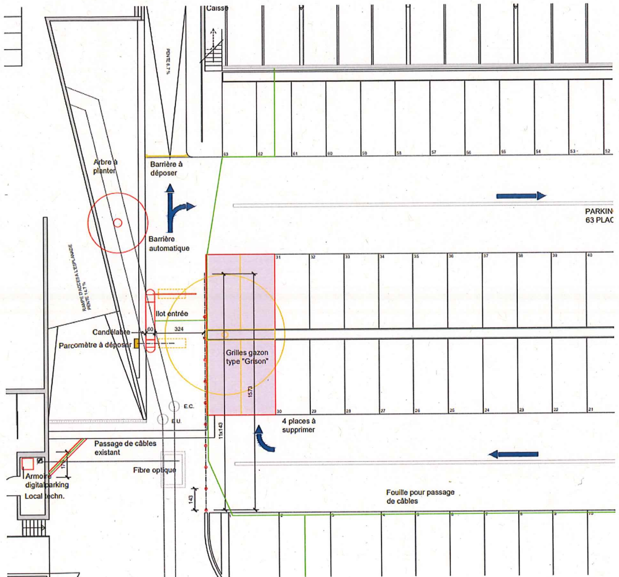
Plan du parking et implantation nouvel arbre
